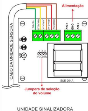
UNIDADE SINALIZADORA
